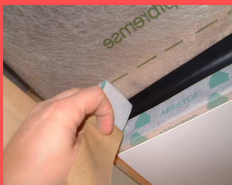
4) Die Manschette wird seitlich mit der Luftdichtungsebene angearbeitet
